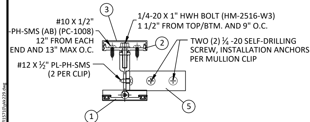
B 2 HORIZONTAL SECTION METAL STUD MULLION CLIP
